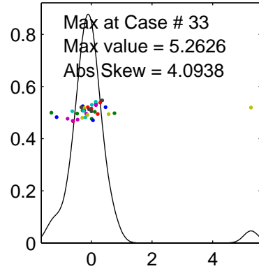
ICA 1 proj., Abs Skew, ir = 6
