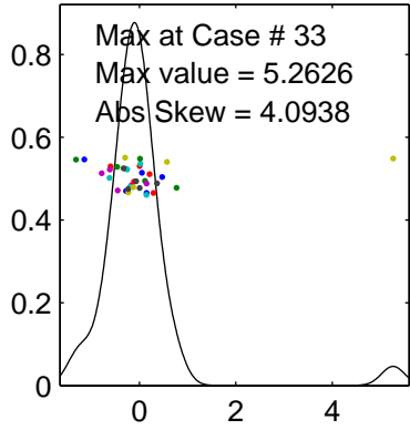
ICA 1 proj., Abs Skew, ir = 5
