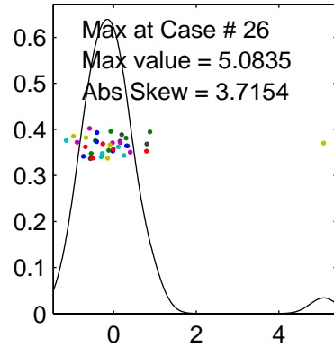
ICA 1 proj., Abs Skew, ir = 10
