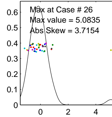
ICA 1 proj., Abs Skew, ir = 8
