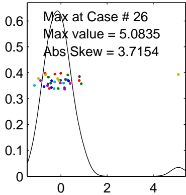
ICA 1 proj., Abs Skew, ir = 9
