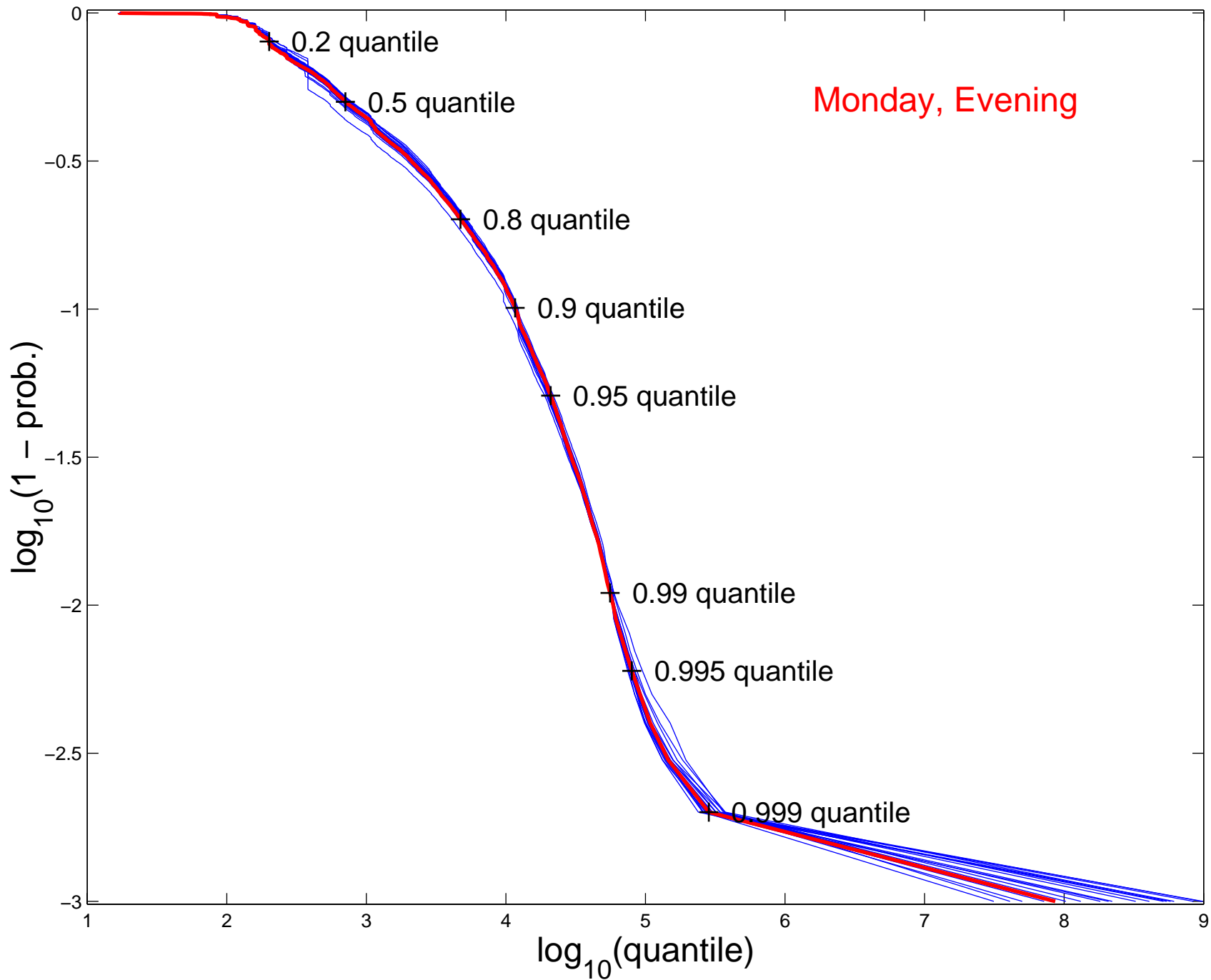
log-log CCDF, HTTP R. S., n = 3575530
