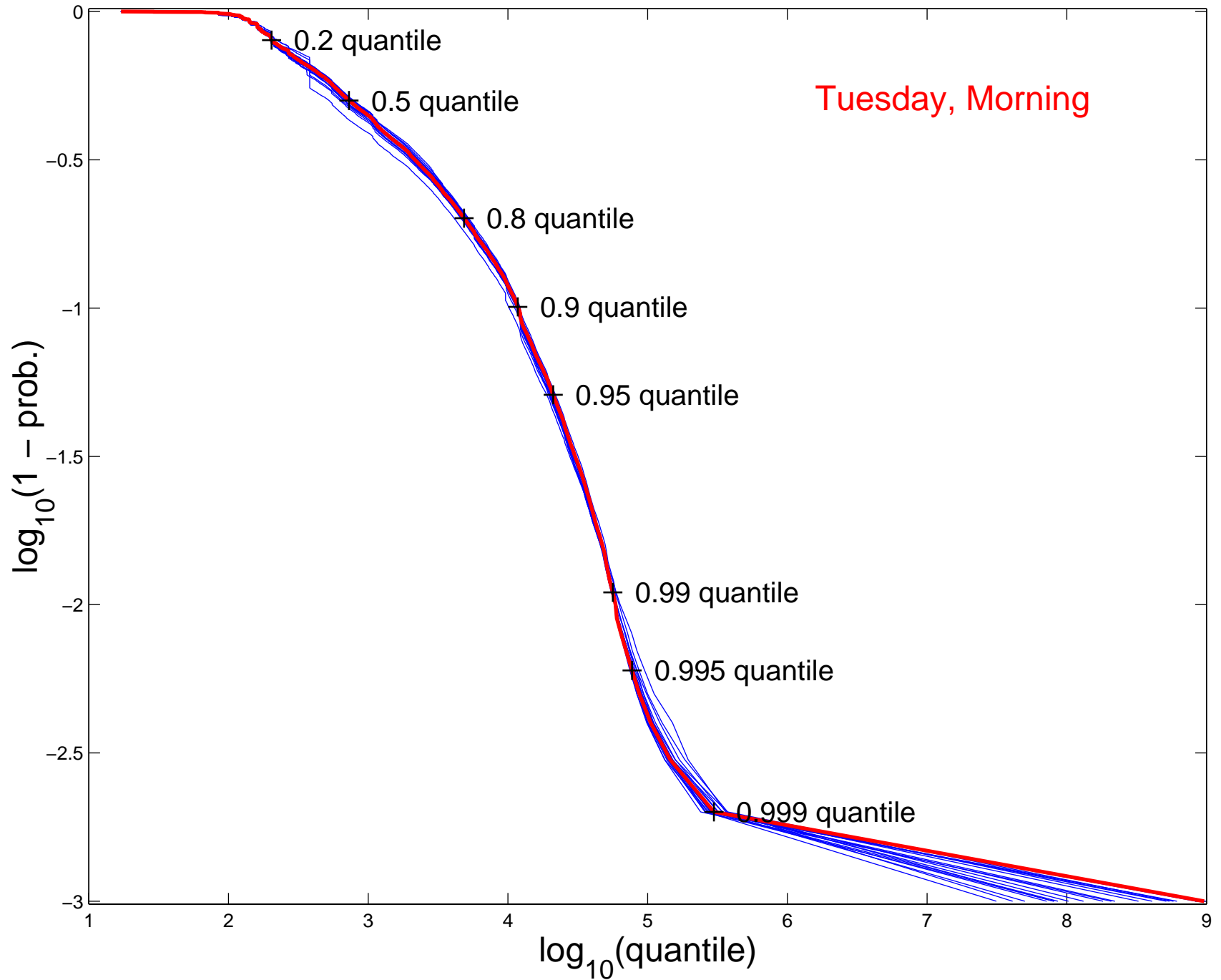
log-log CCDF, HTTP R. S., n = 5614180
