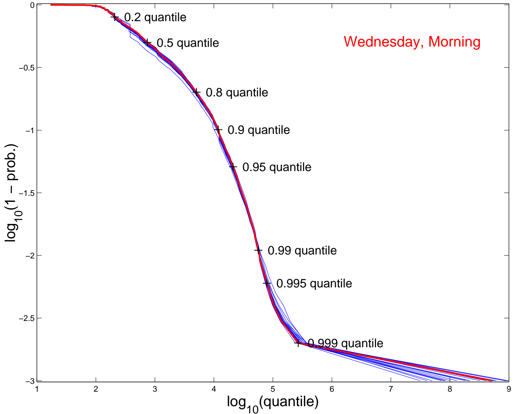
log-log CCDF, HTTP R. S., n = 5625356
