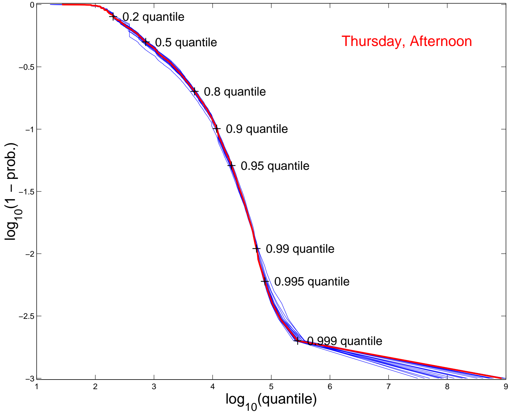
log-log CCDF, HTTP R. S., n = 6870022
