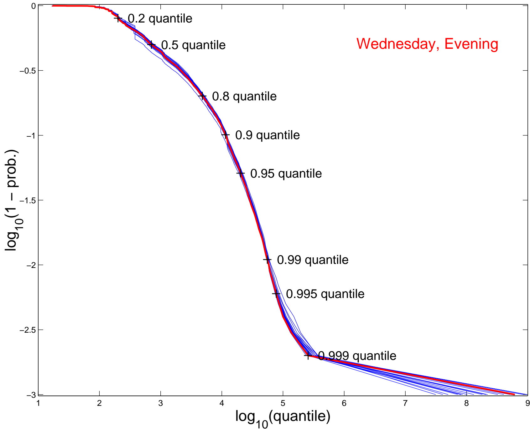
log-log CCDF, HTTP R. S., n = 3703303
