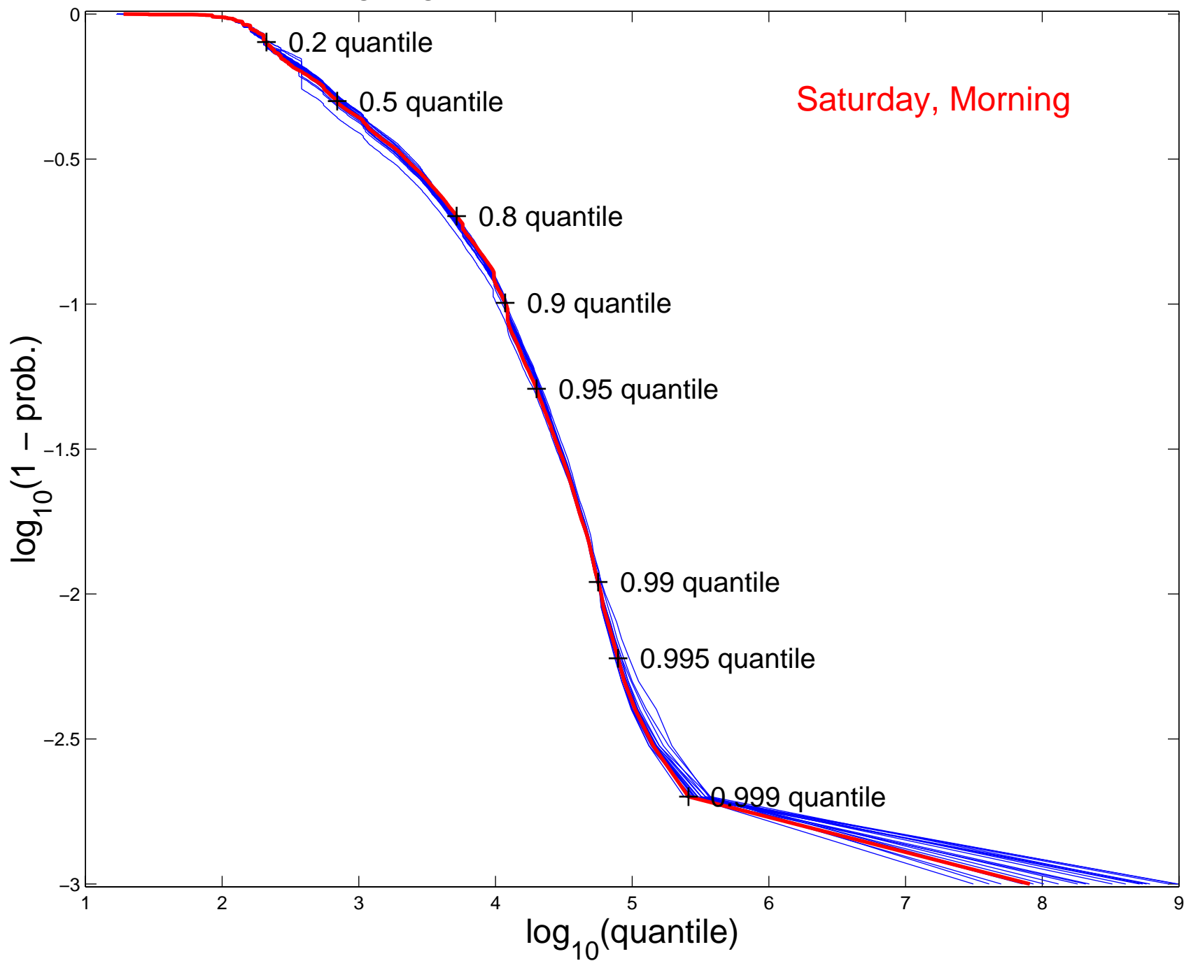
log-log CCDF, HTTP R. S., n = 1187942
