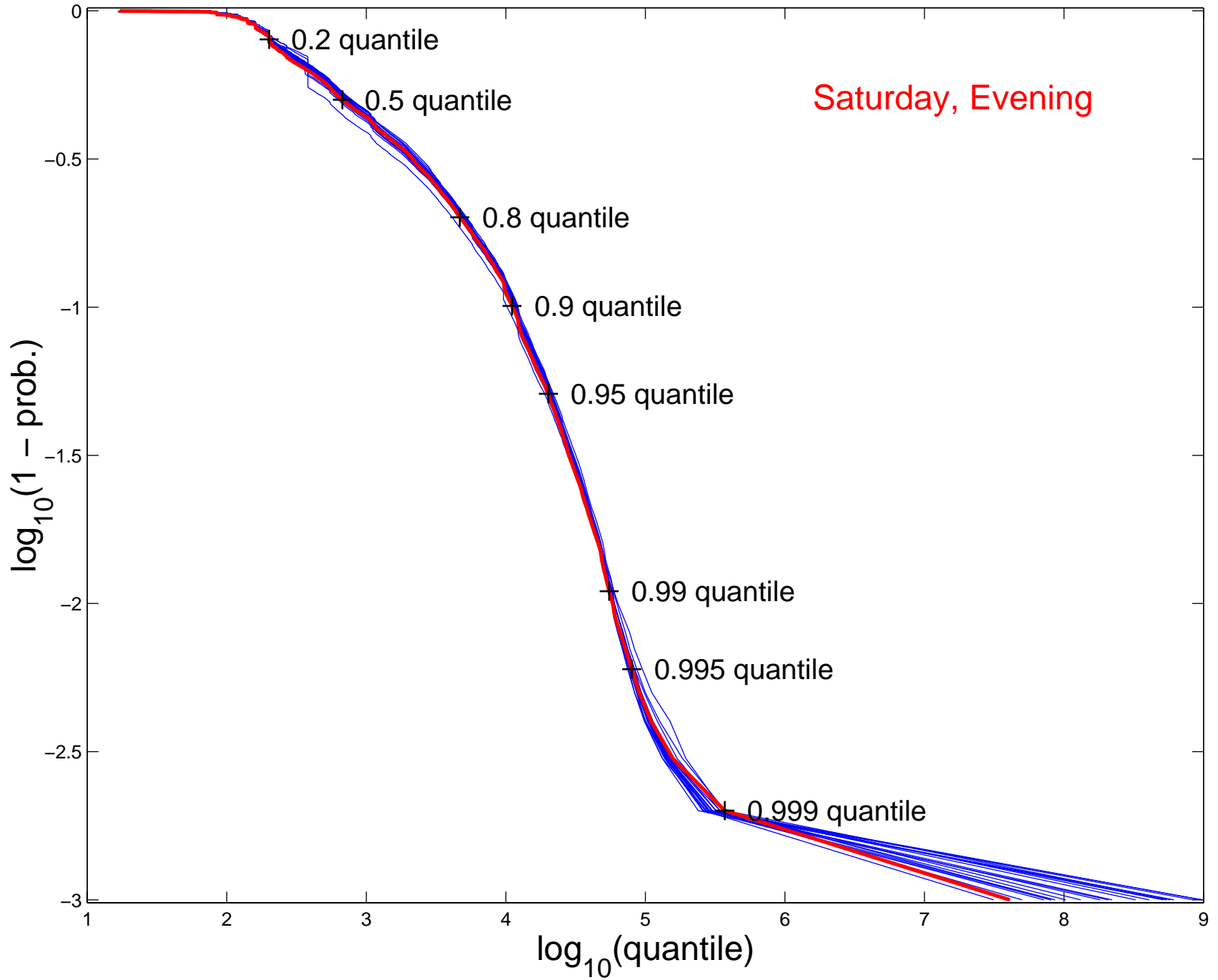
log-log CCDF, HTTP R. S., n = 1843115
