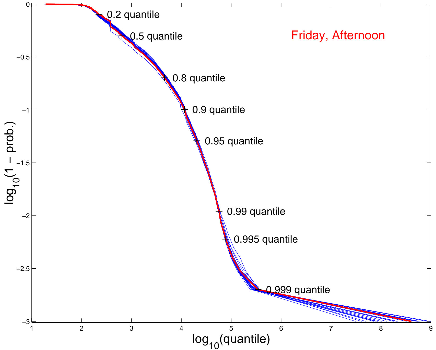
log-log CCDF, HTTP R. S., n = 6353572
