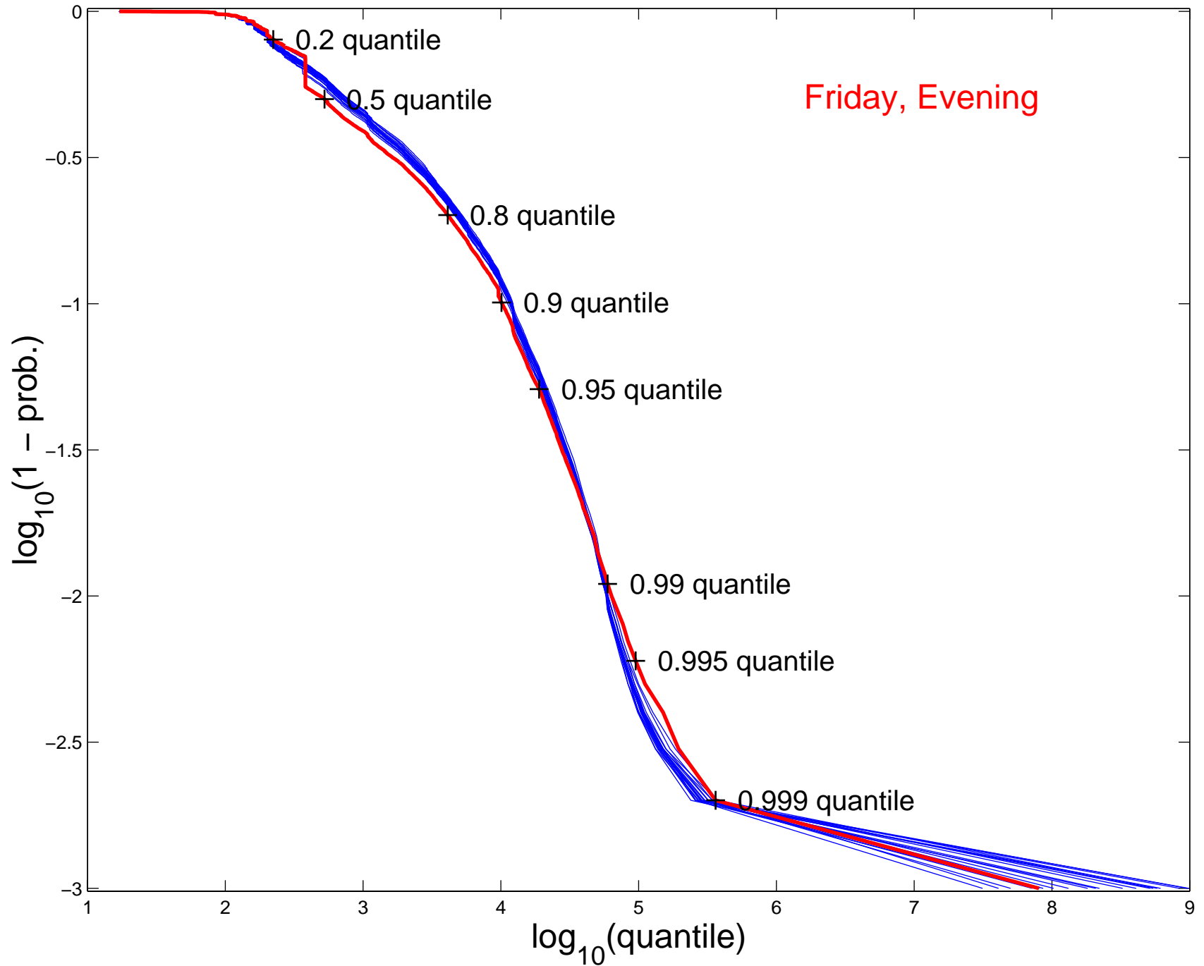
log-log CCDF, HTTP R. S., n = 2087324
