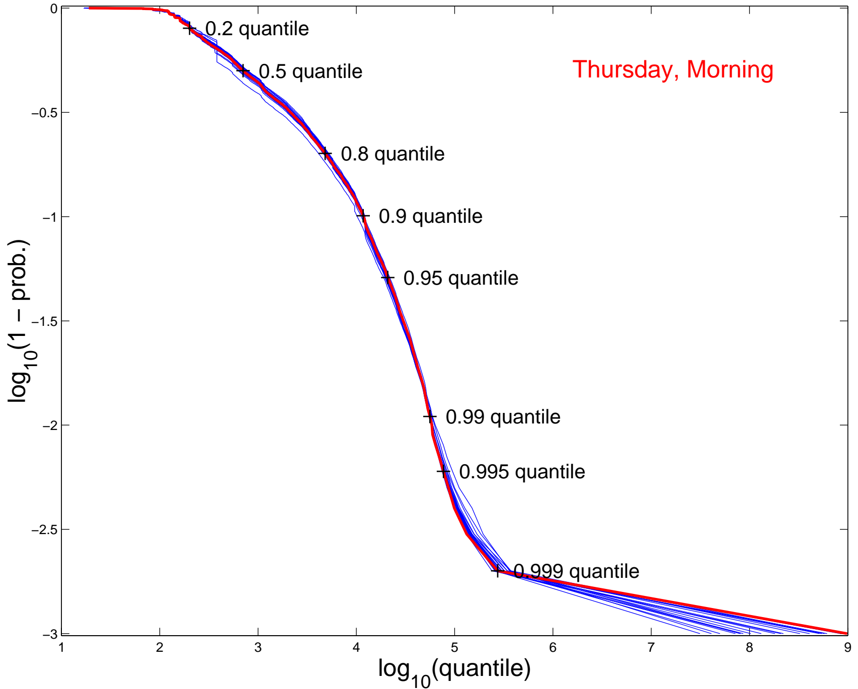
log-log CCDF, HTTP R. S., n = 5663605
