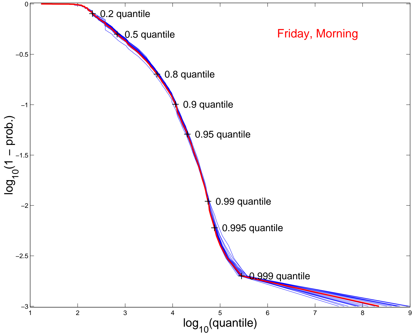
log-log CCDF, HTTP R. S., n = 5326573
