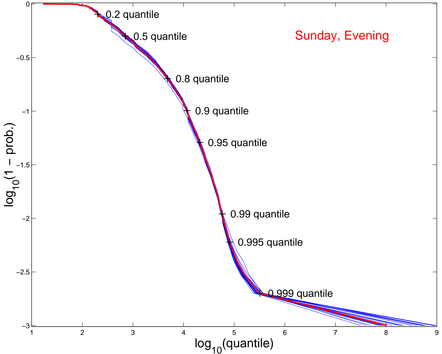
log-log CCDF, HTTP R. S., n = 3147247
