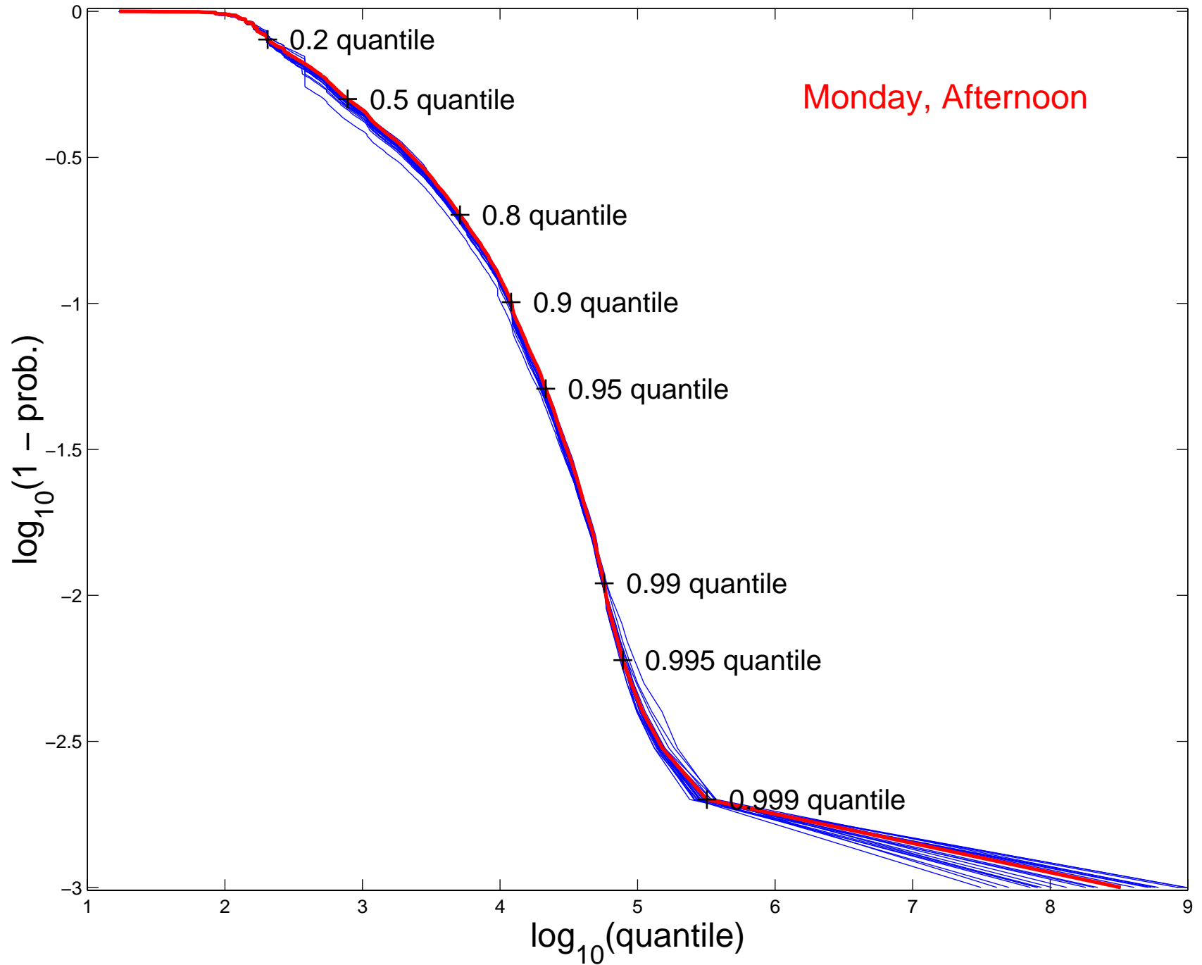
log-log CCDF, HTTP R. S., n = 6935665
