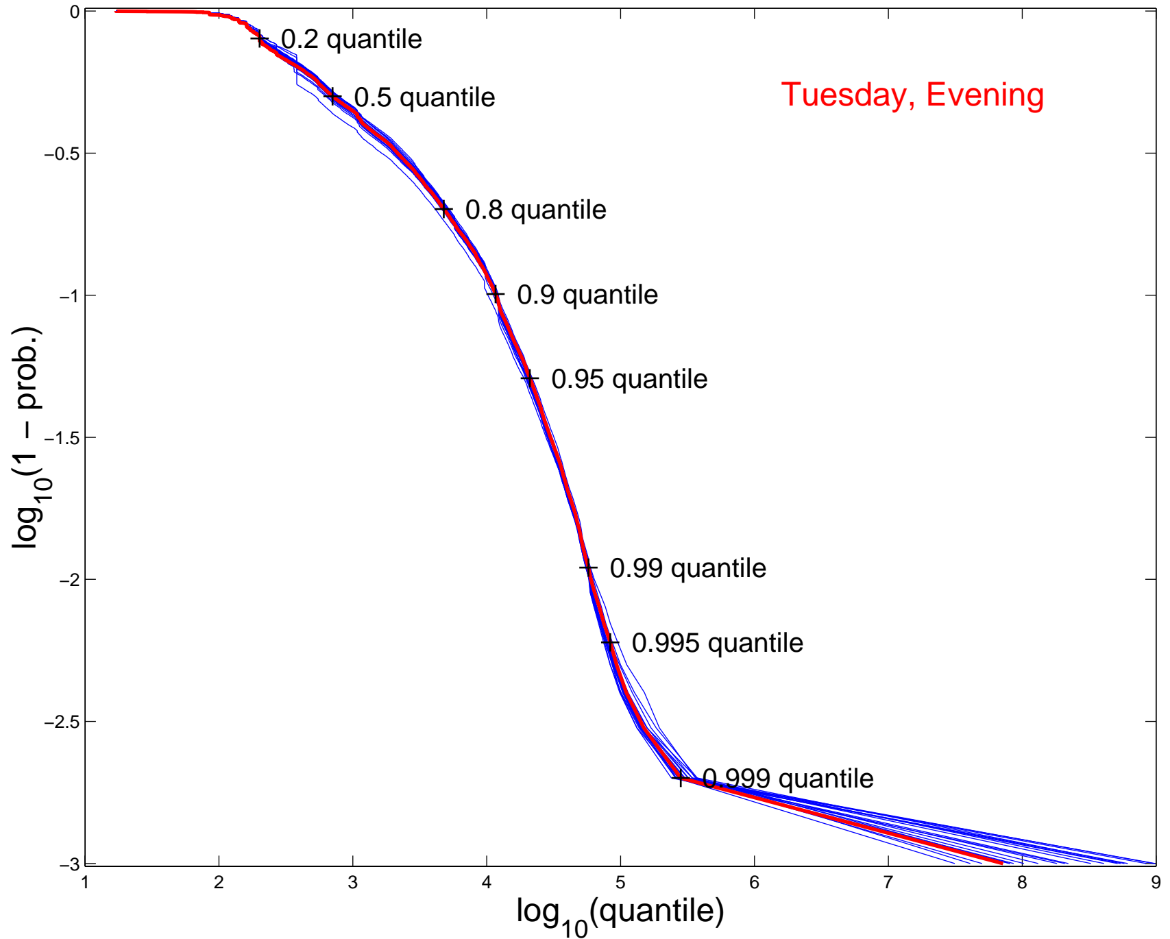
log-log CCDF, HTTP R. S., n = 3525538
