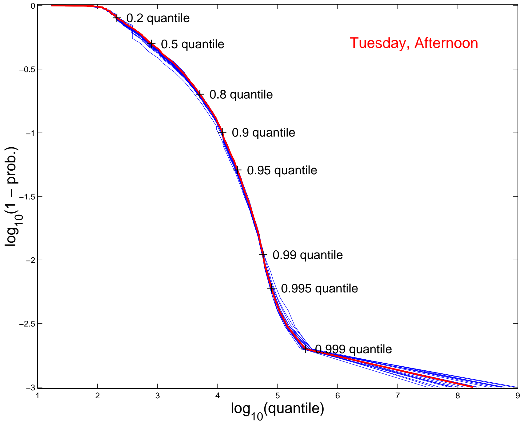
log-log CCDF, HTTP R. S., n = 6763435
