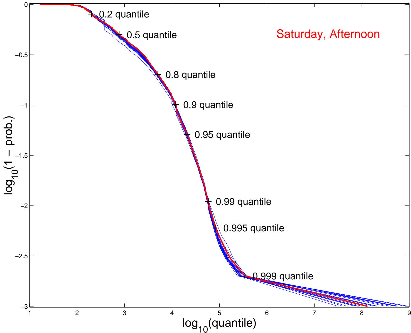
log-log CCDF, HTTP R. S., n = 2638397
