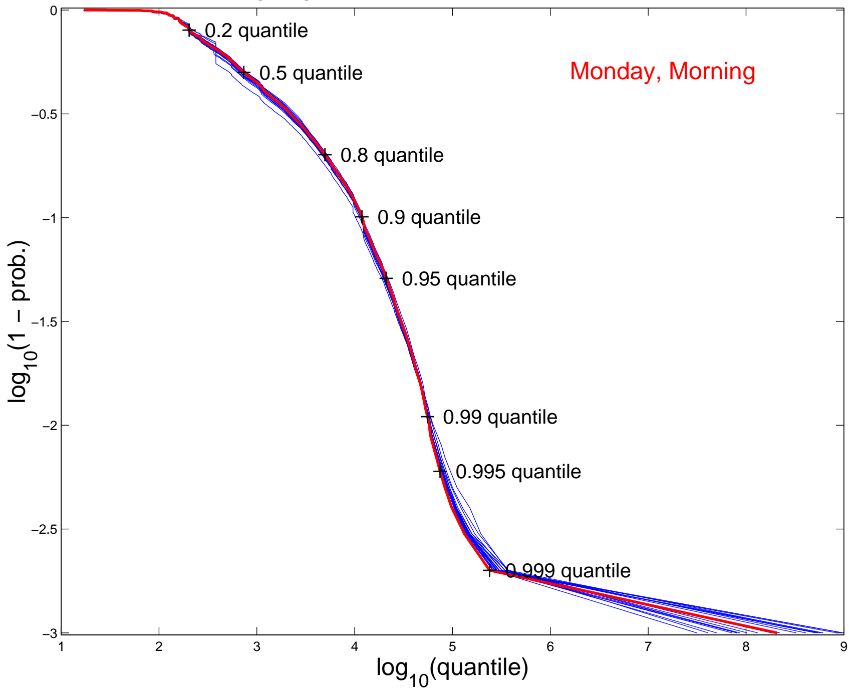
log-log CCDF, HTTP R. S., n = 5621502
