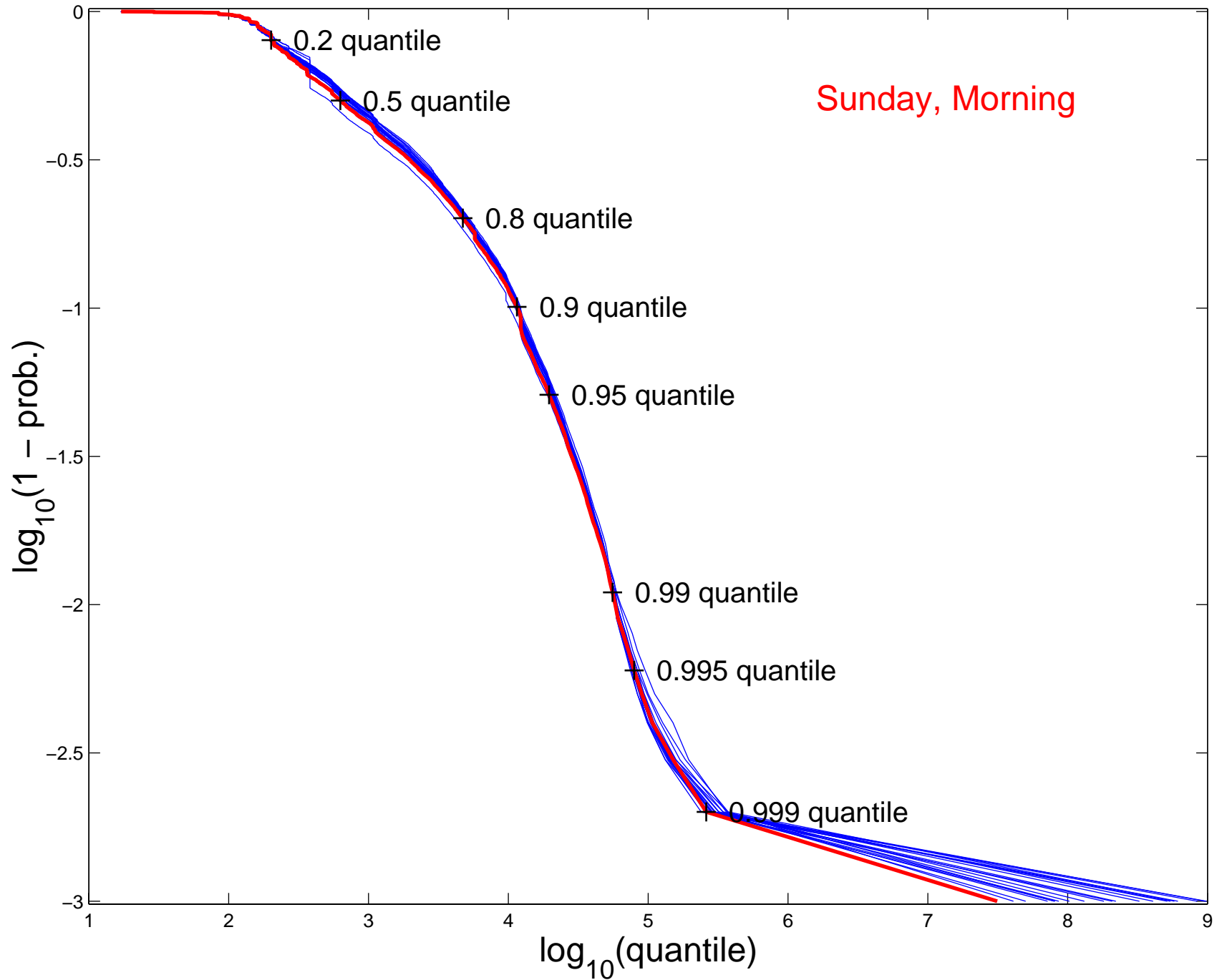
log-log CCDF, HTTP R. S., n = 1070545
