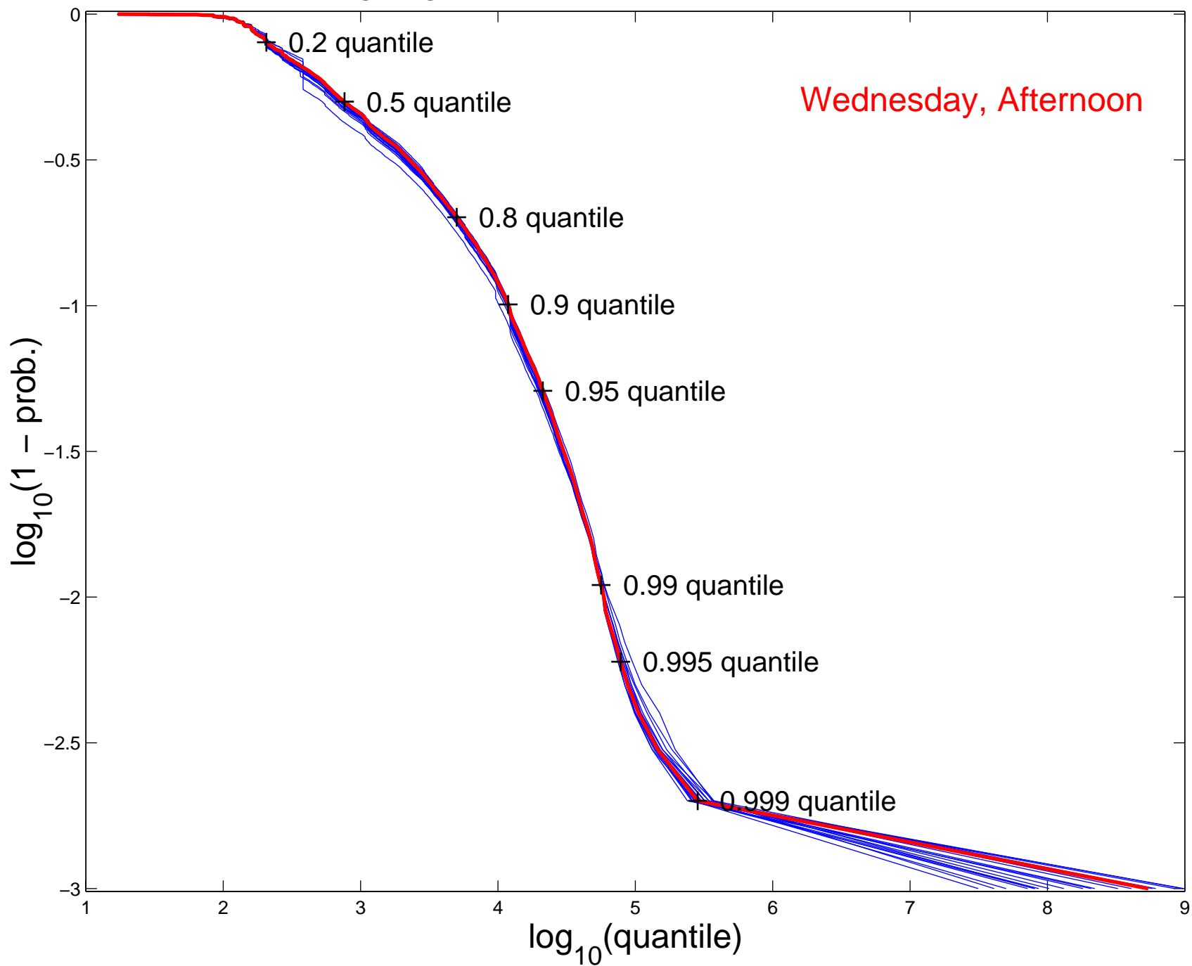
log-log CCDF, HTTP R. S., n = 7136393
