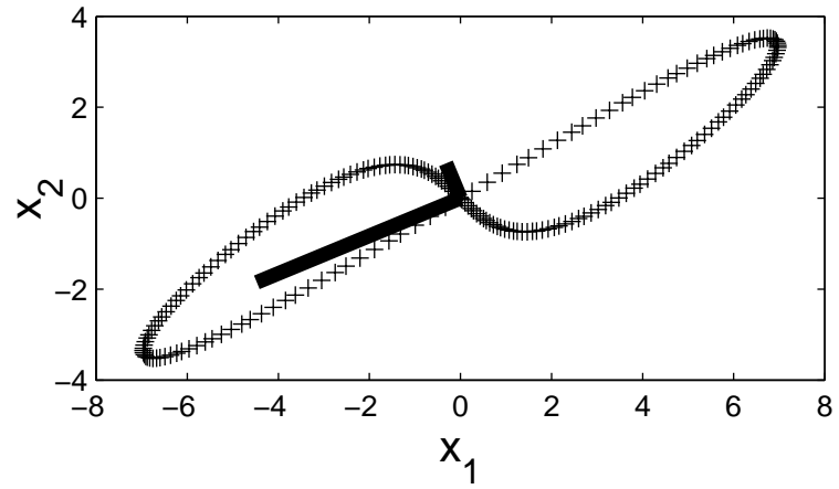
Sin & Sin 2, PCA eigenvectors
